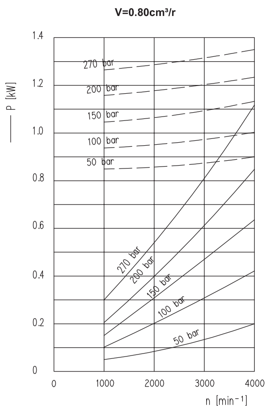
1系列功率性能曲线表/Group 1 Power Performance Curve Table
