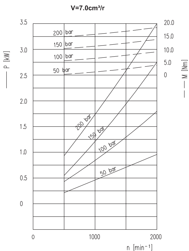
1系列功率性能曲线表/Group 1 Power Performance Curve Table
