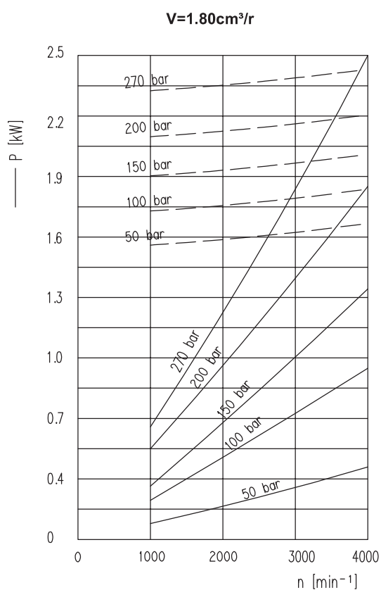
1系列功率性能曲线表/Group 1 Power Performance Curve Table
